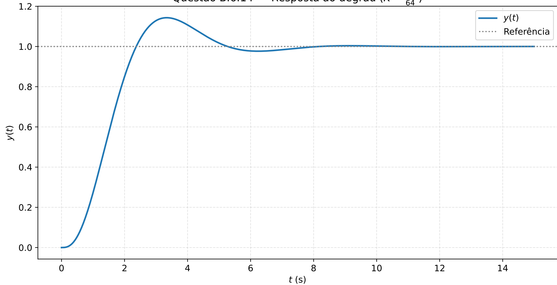
Questão B.6.14 --- Resposta ao degrau ( K = \frac{275}{64} )
